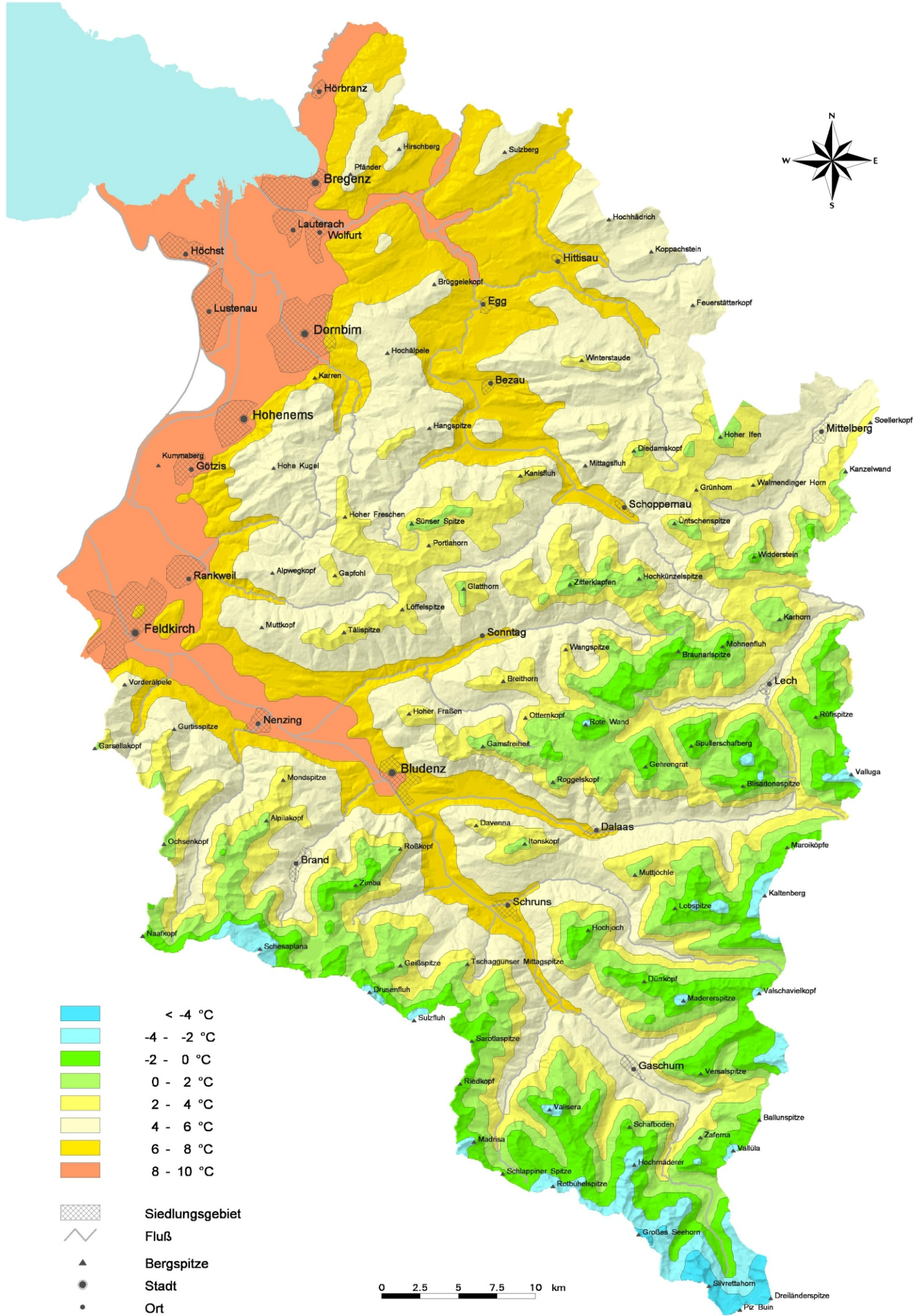
Klima von Vorarlberg Jahresmittel der Lufttemperatur in der Periode 1961 - 1990 Karte 1.1
