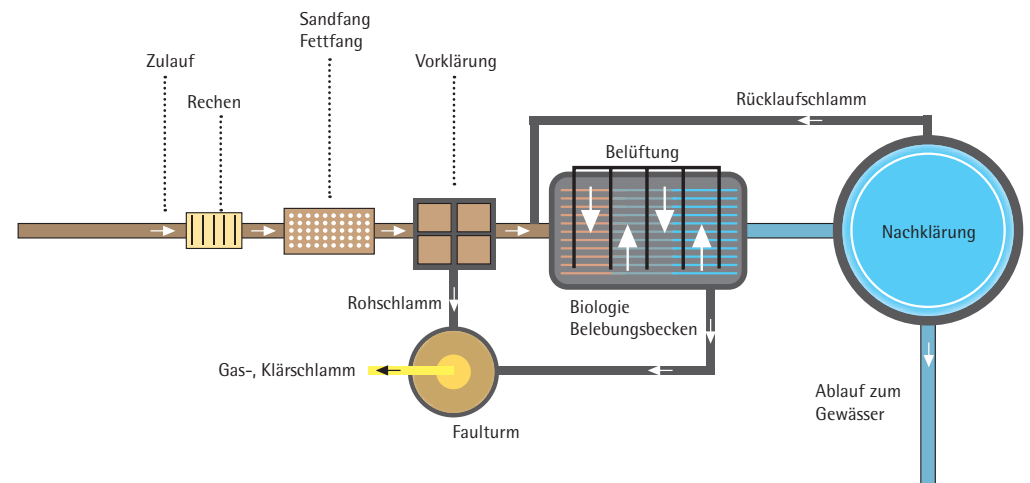
Schema des Reinigungsprozesses in einer Kläranlage
