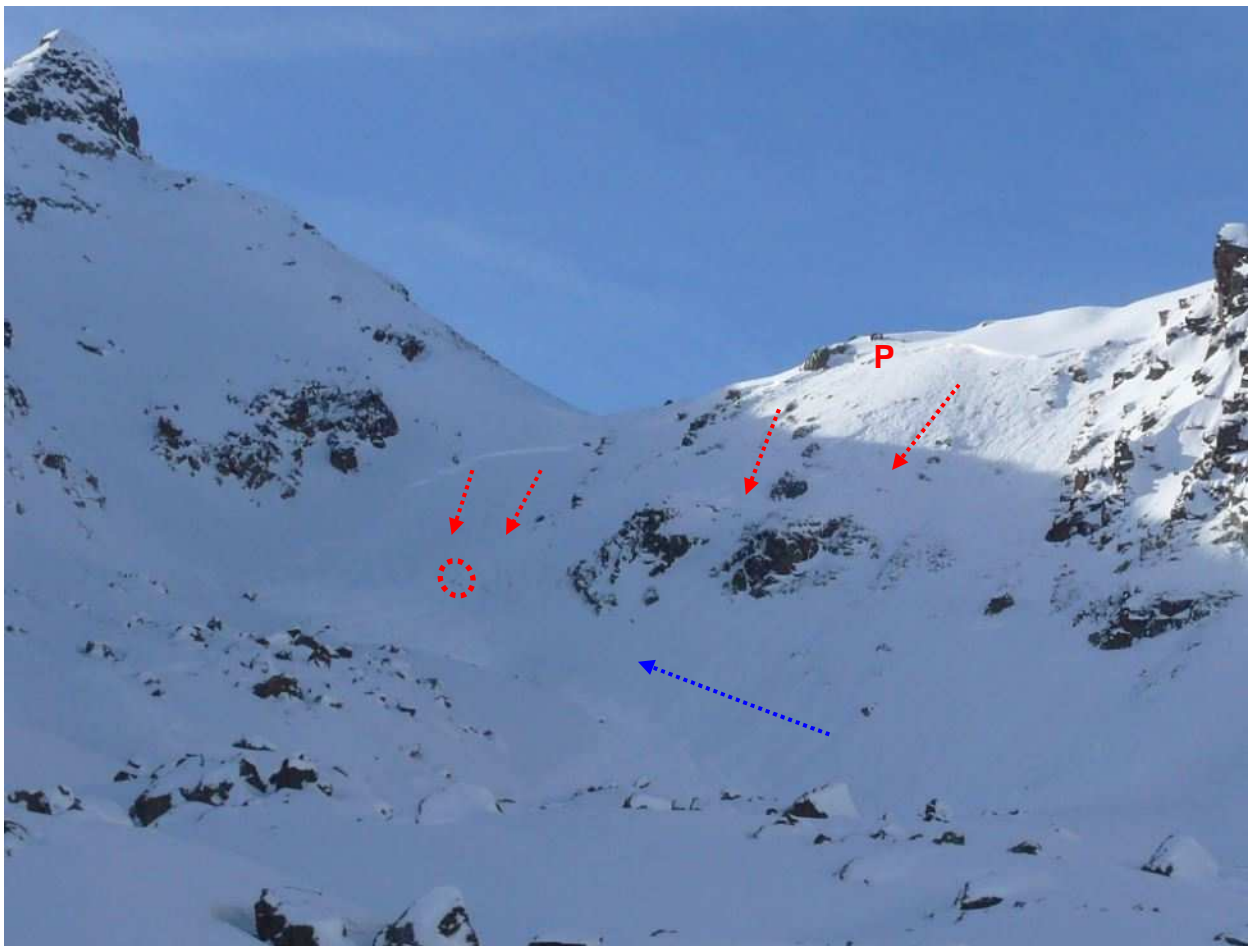
06.01.2015: Geländeübersicht mit ca. Aufstiegsspur (blau), Anrisszone und Ablagerungsbereich sowie den Liegepunkt des verschütteten Wintersportlers (roter Kreis). P = Schneeprofilort – siehe dazu Seite 3
