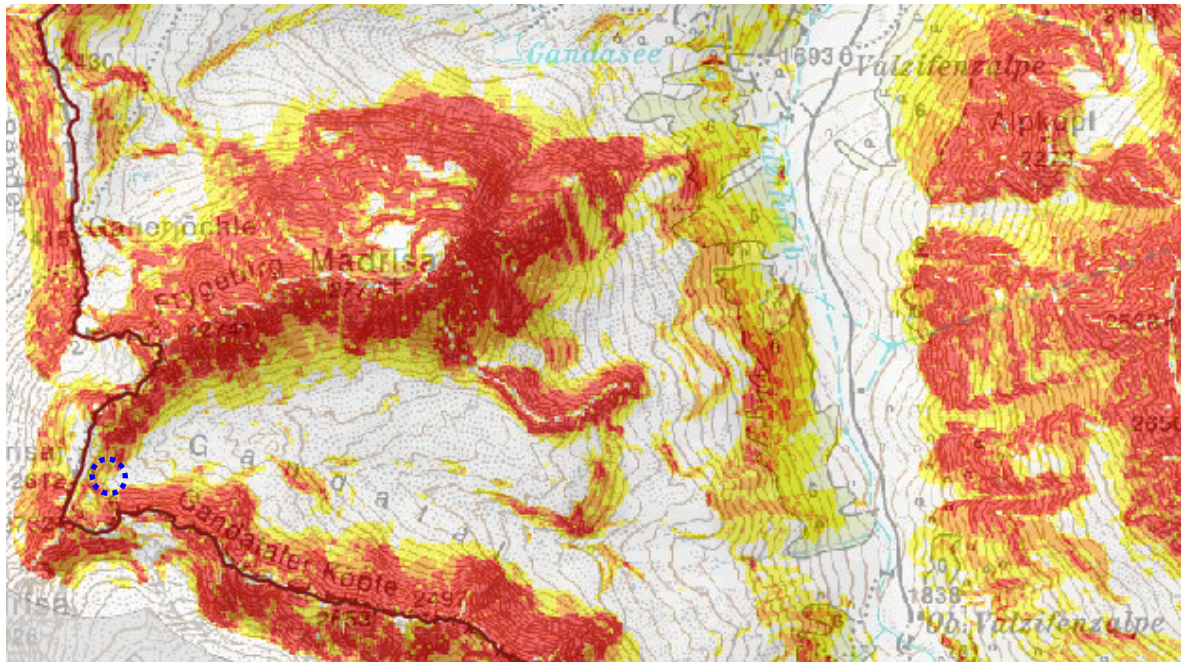
© Hangneigungskarte: Vogis, LVA Feldkirch: Übersicht mit Hangneigungen und ca. Ereignisbereich (blau)
